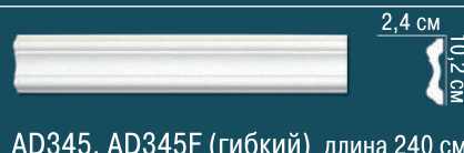
AD345, AD345F (гибкий) длина 240 см
