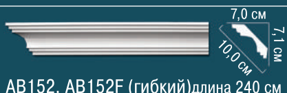
AV152, AV152F (гибкий) длина 240 см
