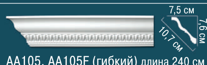
AA105, AA105F (гибкий) длина 240 см
