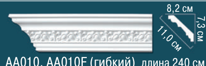
AA010, AA010F (гибкий) длина 240 см
