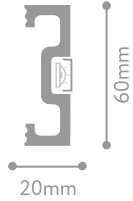
2UHD 10/60L Рассеиватель в комплекте
